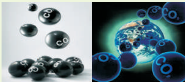
OZONE IN DYNAMIC BALANCING O_3 = O_2 + O = O_3
