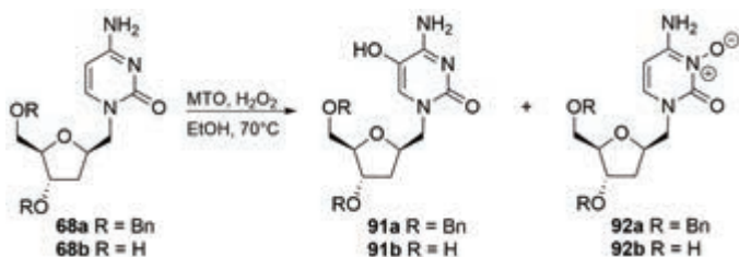
Schemat 14. Utlenienie 3',5'-di-O-benzyl-1'-homo-2'-deoksytydyny 68a
