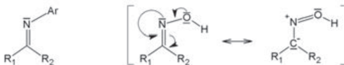
Rysunek 3. Struktura imin stabilizowana podstawnikiem aryłowym oraz elektrodonorowym Figure 3. The structure of imines stabilized aryl and electro donor chemical entity
