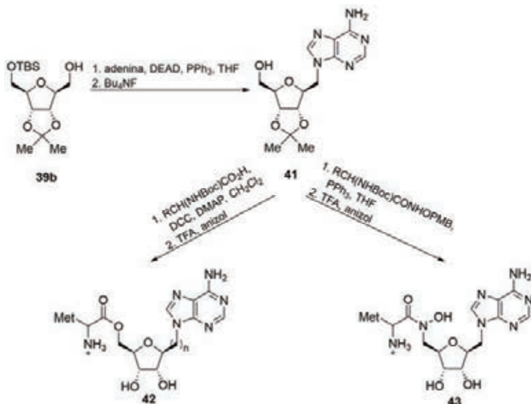
Schemat 8. Synteza analogów 1'-homonukleozydów jako potencjalnych inhibitorów syntetazy metionyl- t -RNA 42 i 43
