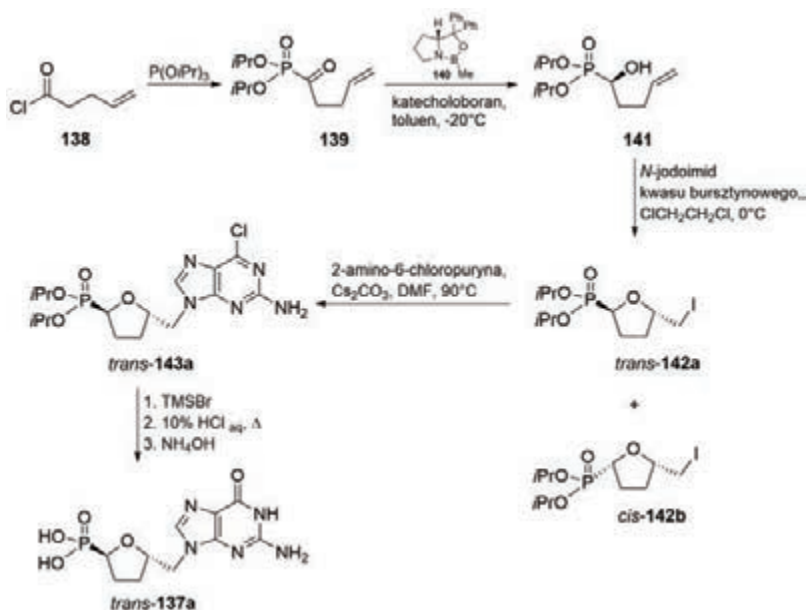
Schemat 23. Fosfonanowe analogi 1'-homonukleozydów trans -137a i trans -143a
