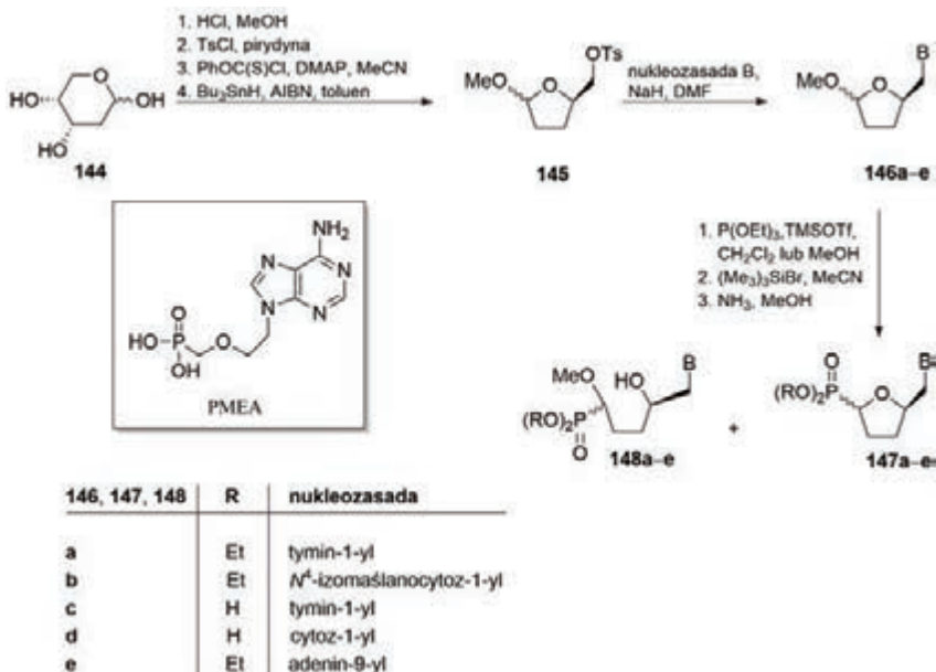
Schemat 24. Synteza fosfonianowych analogów 1'-homonukleozydów 147a-e
