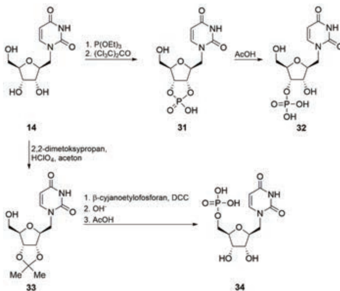
Schemat 6. Synteza fosforanowych pochodnych 1'-homourydyny 32 i 34
