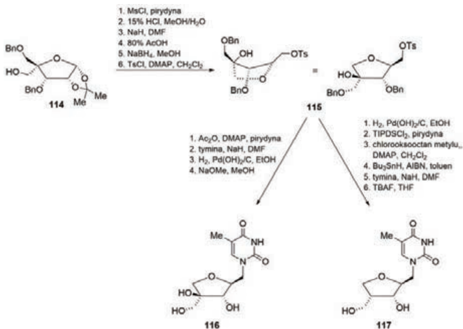
Schemat 19. Synteza LNA 1'-homonukleozydów 116 i 117
