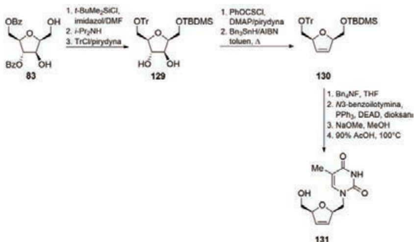
Schemat 21. Synteza 1'-homostawudyny 131
