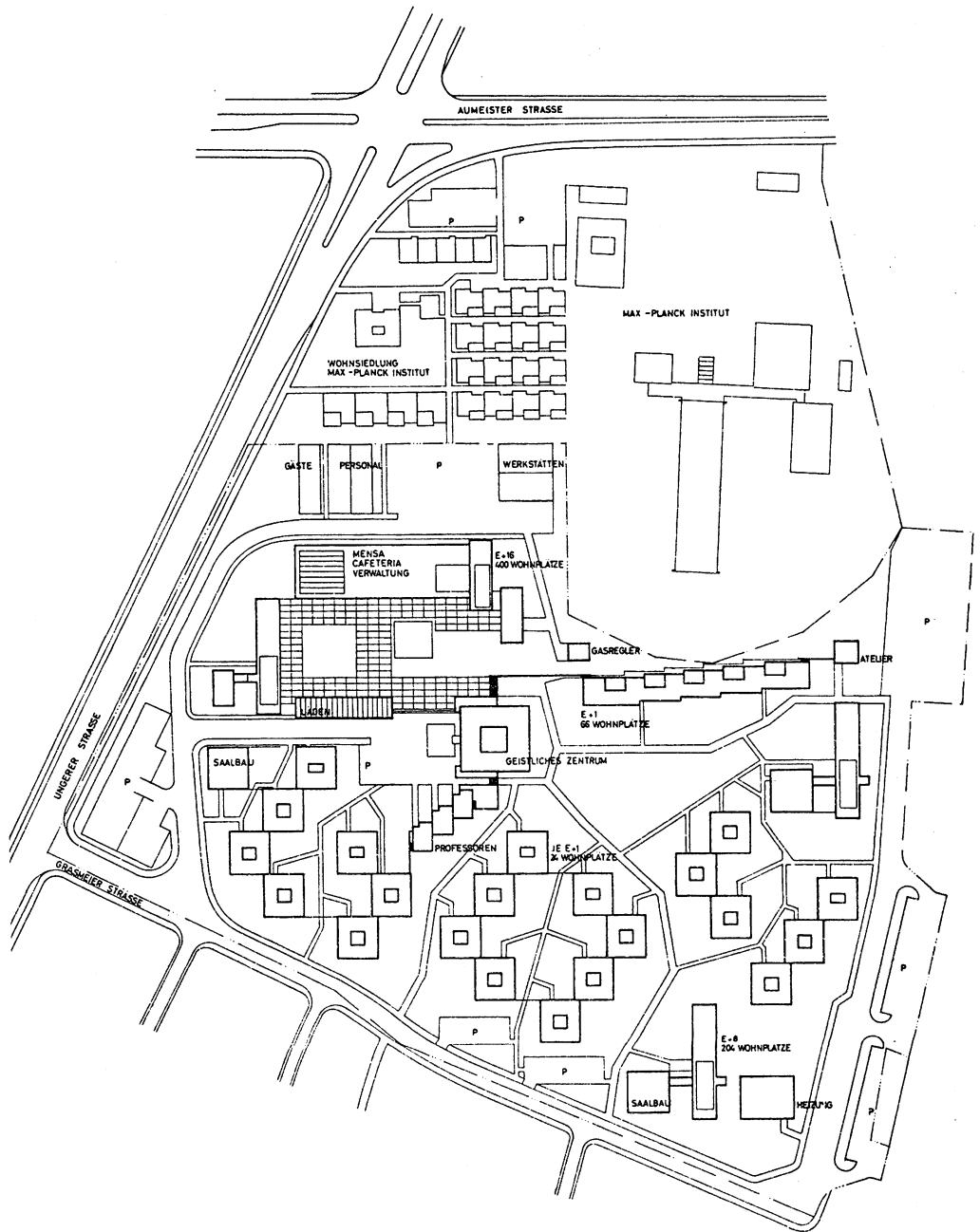
Lageplan der Studentenstadt München
