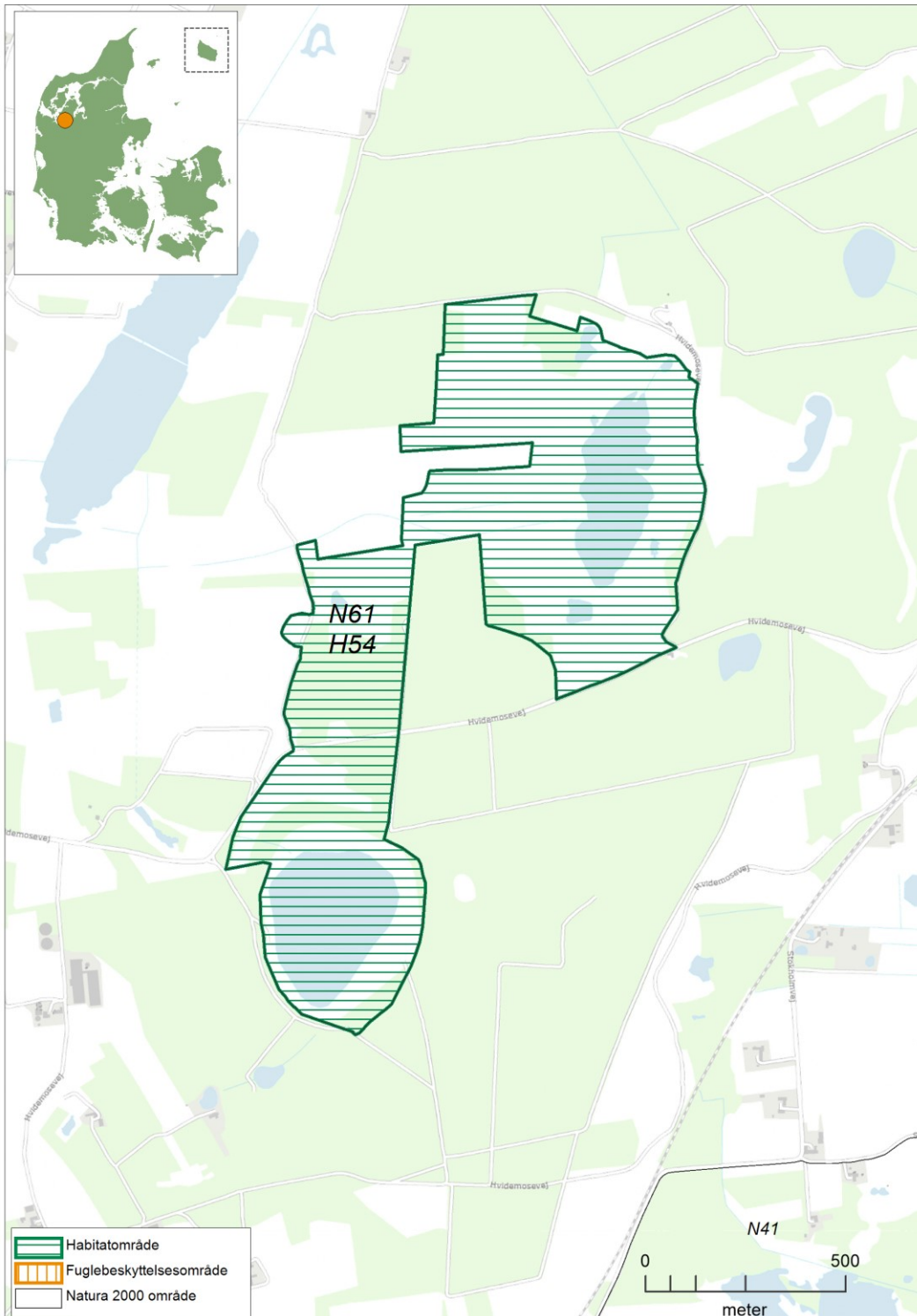
Kortet viser Natura 2000-områdets afgrænsning. Natura 2000-område N61 Skånsø og Tranemose består af habitatområde H61 Skånsø og Tranemose (vandret grøn skravering).
