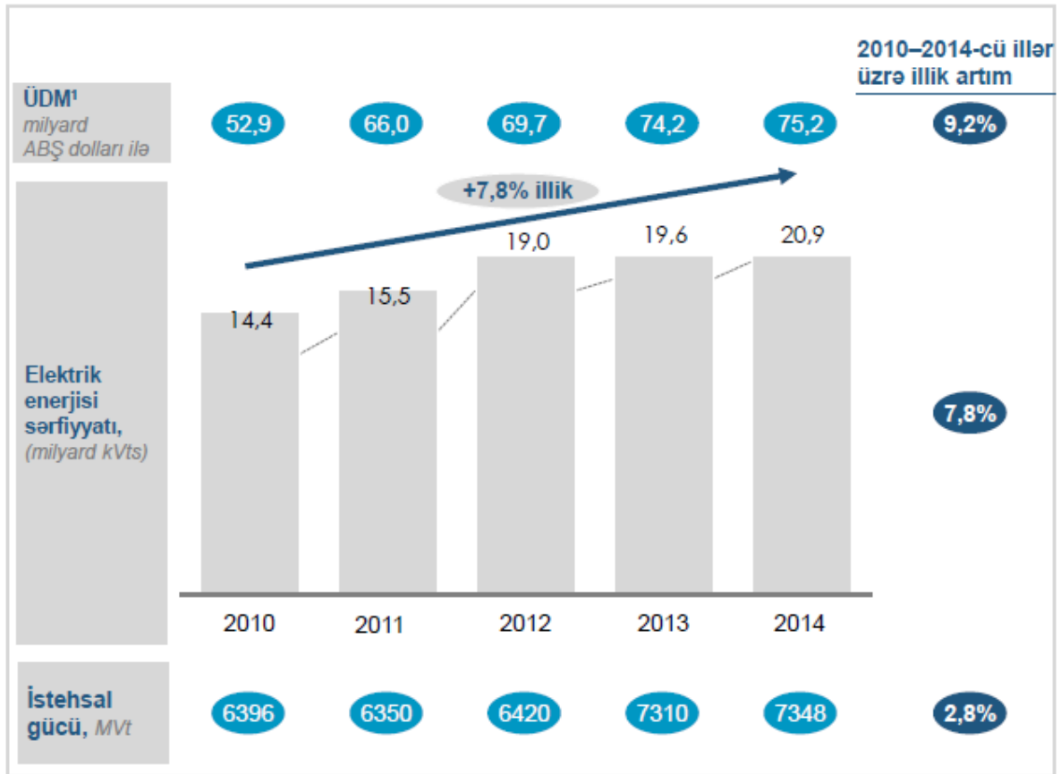
Diaqram 3. Elektrik enerjisi istehlakının ÜDM-ə paralel olaraq artımı
