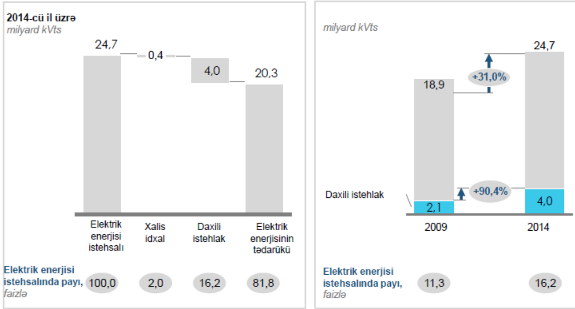
Diaqram 11. Elektrik stansiyalarında elektrik enerjisindən daxili istifadə
