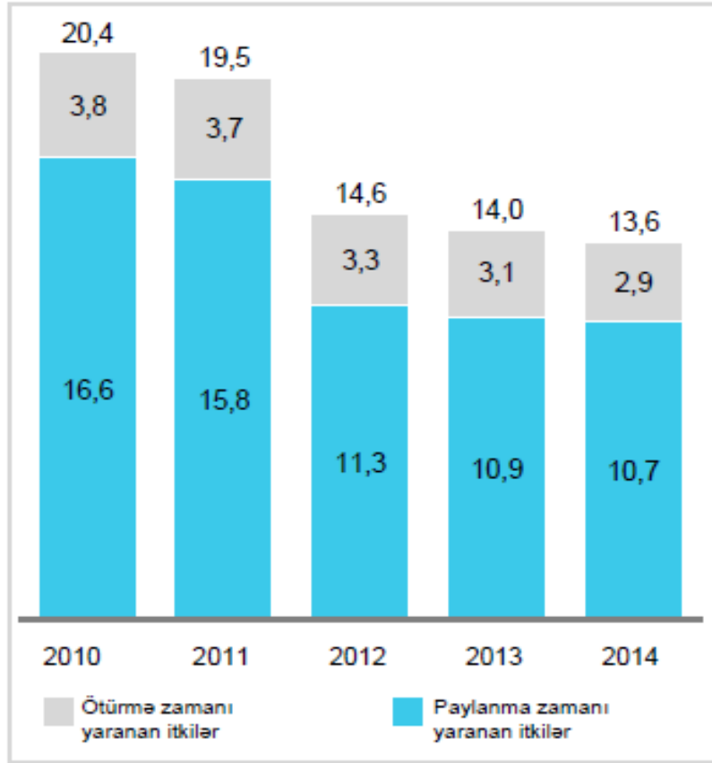
Diagram 14. Elektrik enerjisinin ötürülməsi və paylanması üzrə itkilər (faizlə)
