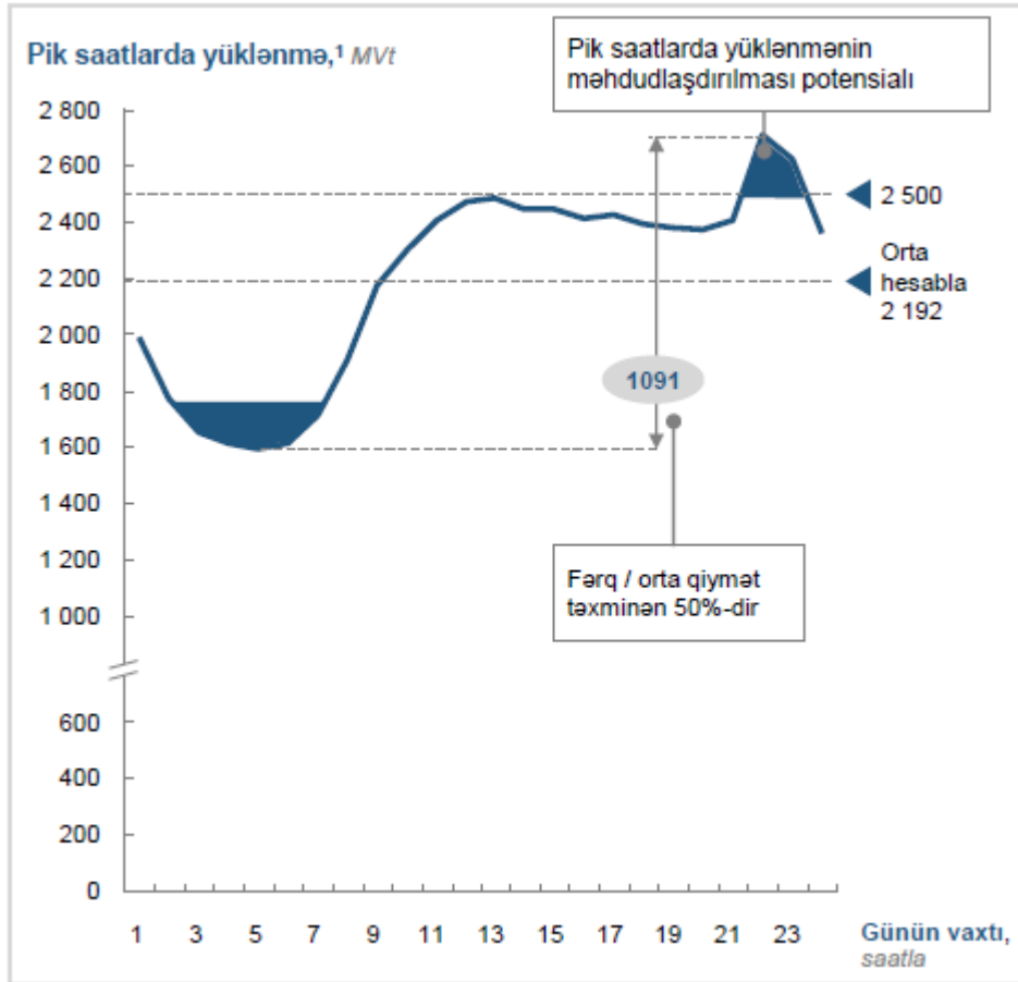
Qrafik 3. Gecə-gündüz tariflərinin gündəlik yük göstəricilərinə təsiri
