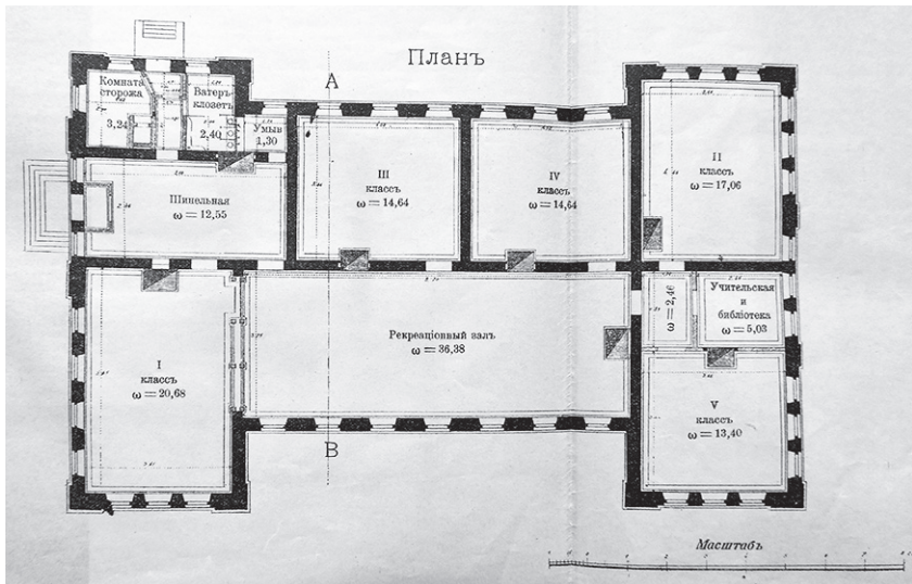
План будівлі Слов'янської 2-х класної залізничної школи
