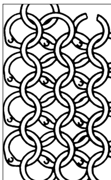
Схема плетіння кольчуги зі зварених і склепаних кілець.
