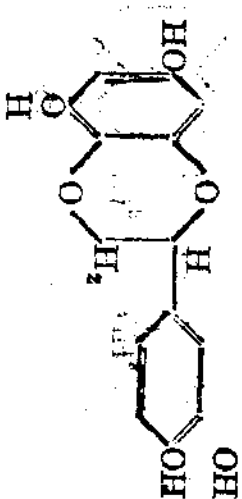
(維生素P的構造式)
