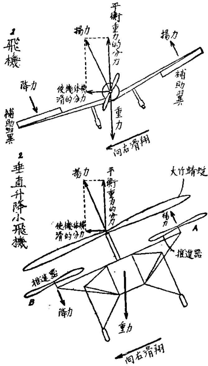
圖 2. 垂直升降小飛機側傾原理圖 (從正面直視)
