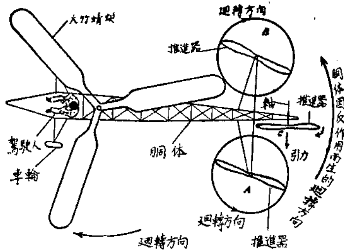
圖1. 希科耳斯基式垂直升降小飛機飛翔原理圖 (從上方俯視)
