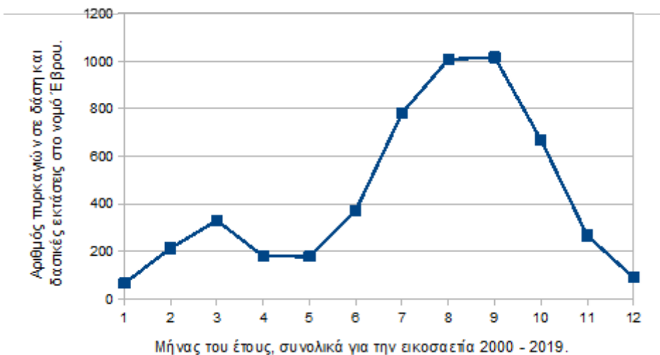
Διάγραμμα 7. Αριθμός πυρκαγιών σε δάση και δασικές εκτάσεις σε σχέση με τον μήνα του έτους.
