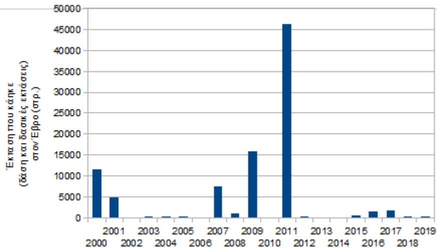
Διάγραμμα 1. Η καμένη επιφάνεια ανά έτος (δάση και δασικές εκτάσεις) στον Έβρο την εικοσαετία 2000-2019.
