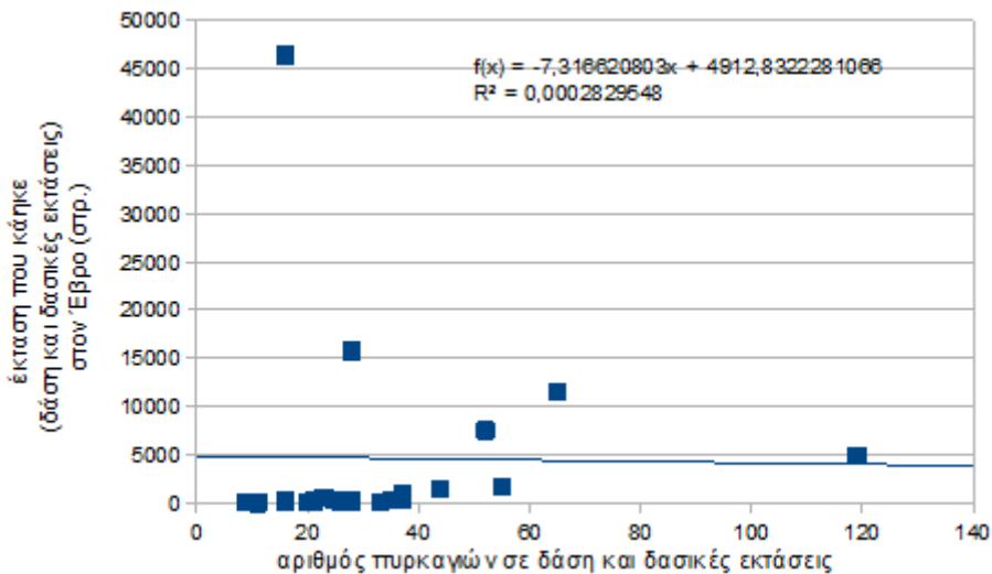
Διάγραμμα 6. Συσχέτιση καμένης έκτασης με τον αριθμό πυρκαγιών στο νομό Έβρου την εικοσαετία 2000-2019.
