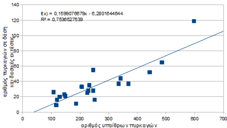
Διάγραμμα 5. Συσχέτιση αριθμού πυρκαγιών σε δάση και δασικές εκτάσεις με τον συνολικό αριθμό υπαίθριων πυρκαγιών στο νομό Έβρου την εικοσαετία 2000-2019.
