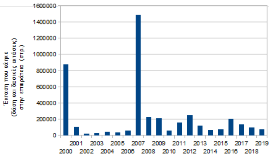
Διάγραμμα 2. Καμένη επιφάνεια (δασών και δασικών εκτάσεων) στην Ελληνική επικράτεια την εικοσαετία 2000-2019.
