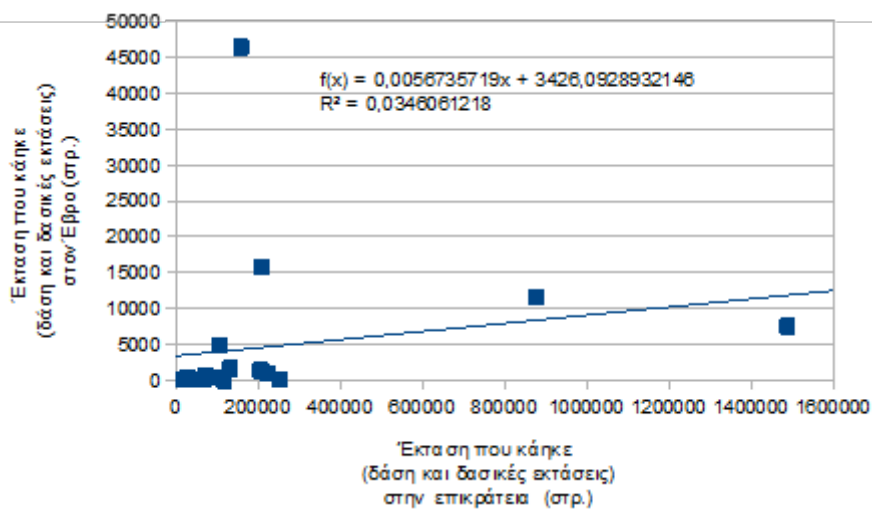
Διάγραμμα 3. Συσχέτιση καμένης έκτασης στον Έβρο και την επικράτεια.
