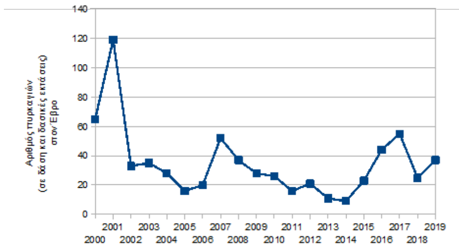
Διάγραμμα 4. Αριθμός πυρκαγιών σε δάση και δασικές εκτάσεις στον Έβρο την εικοσαετία 2000-2019.
